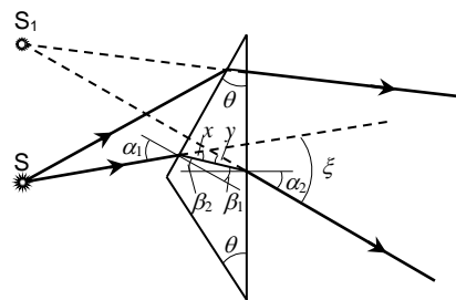
6.2 pav. Spindulių nuokrypis biprizmėje
