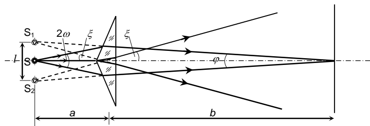
6.3 pav. Koherentinių bangų sukūrimas biprizme
