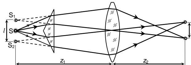
6.4 pav. Atstumo tarp tariamųjų spinduolių nustatymo schema
