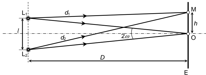
6.1 pav. Bendroji bangų interferencijos schema
